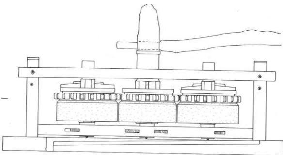
黒砂糖搾り機(側面図)
